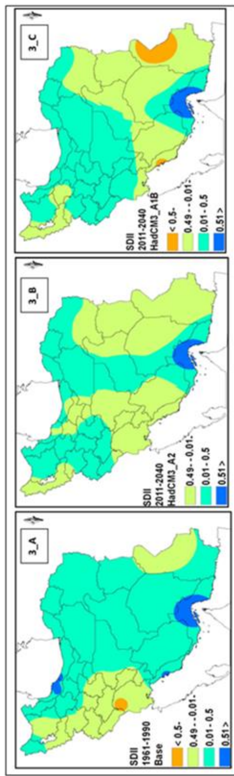
شکل ۳. روند خطی نمایه‌ی سادگی شدت روزانه بر حسب میزان آن بر دهه‌ی پایه (۱۹۶۱-۱۹۹۰) و دوره‌ی آتی (۲۰۱۱-۲۰۴۰).
