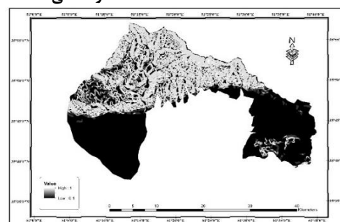
شکل ۷. فازی سازی طبقات شیب.
