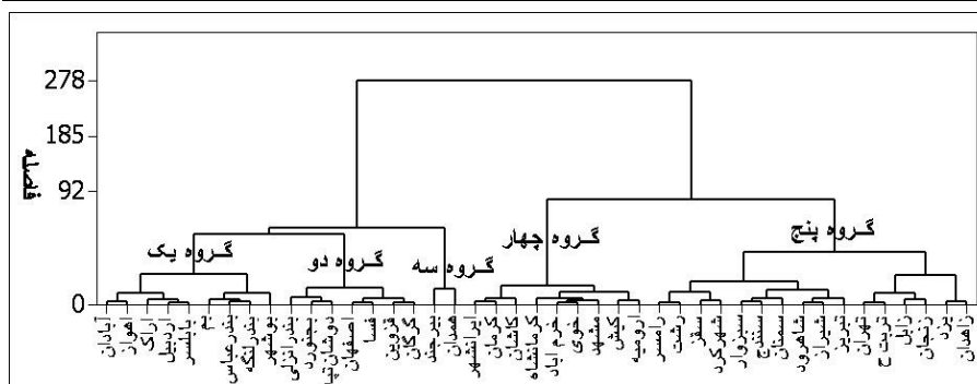
شکل (۲) نمودار شاخه‌درختی خوشه‌بندی ایستگاه‌ها بر مبنای مجموع درصد رده‌های خشکسالی
