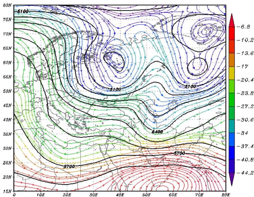
شکل (۷) نقشه های ترکیبی ارتفاع ژئوپتانسیل و فرارفت دمای تراز ۵۰۰ هکتوپاسکال در ساعت صفر Z روز ۱ فوریه ۱۹۹۷
