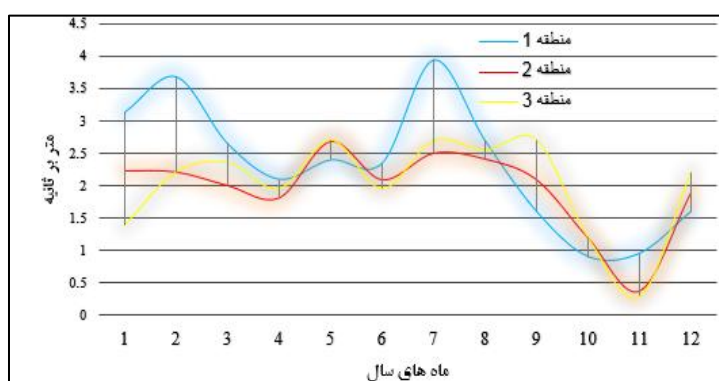
شکل (۱۲). میانگین سرعت باد در ماه های مختلف
