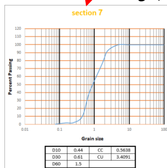
د- منحنی دانه بندی از نقطه ۷، بازه مکانی ۵
