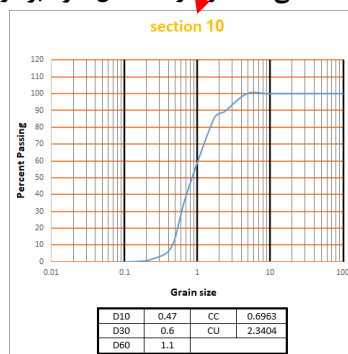
ج- منحنی دانه بندی از نقطه ۱۰، بازه مکانی ۳
