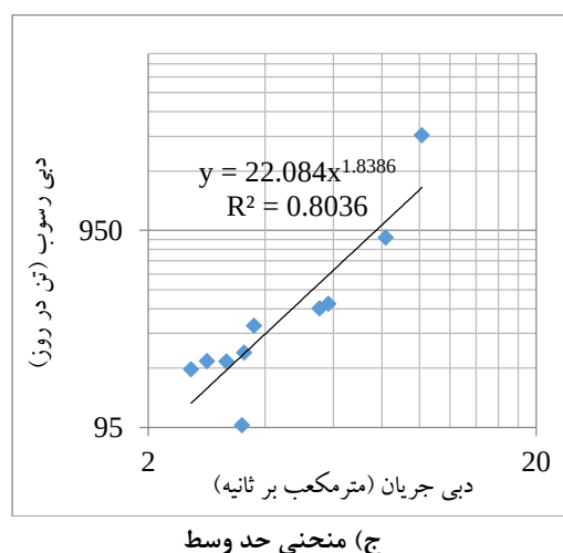
شکل (۱۱). نتایج انتخاب منحنی رسوب براساس معادلات یک به یک در ایستگاه شیرگاه
