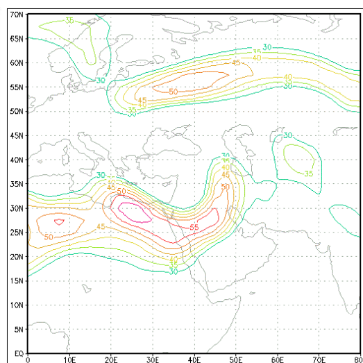
شکل (۱۹). نقشه روداد تراز ۳۰۰ در ۱ آوریل ۲۰۱۹
