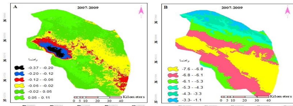
شکل (۳): (A)، دامنه فرونشست منطقه با استفاده از تصاویر سنجنده ASAR (m)، (B): درونابی سطح آبهای زیرزمینی با استفاده از آمار چاه‌های پیزومتر (cm)
