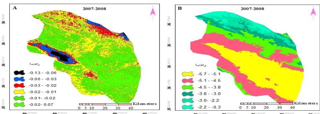
شکل (۴): (A)، دامنه فرونشست منطقه با استفاده از تصاویر سنجنده ASAR (m)، (B): درونابی سطح آبهای زیرزمینی با استفاده از آمار چاه‌های پیزومتر (cm)
