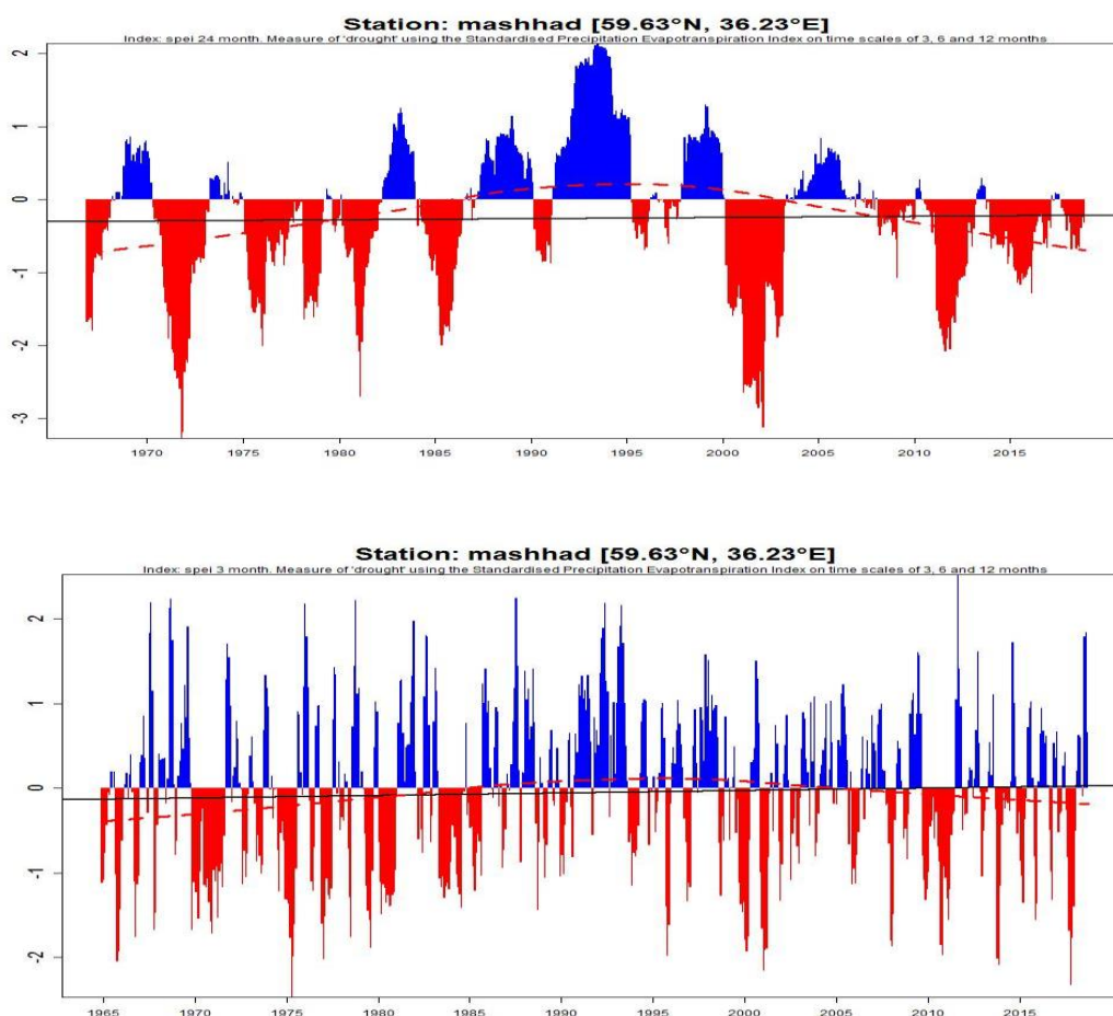
شکل (۱۱): نمودار خشکسالی بر اساس شاخص spei-3-24
