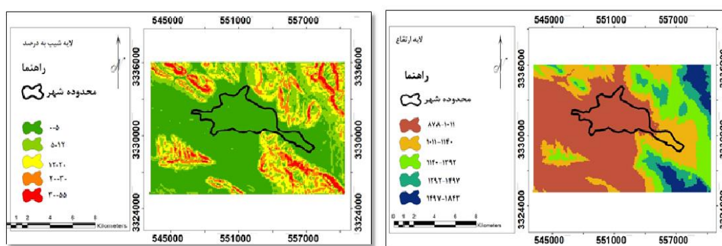
شکل (۲). لایه ارتفاع و شیب محدوده مورد مطالعه
