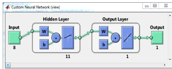
شکل (۴). ساختار شبکه عصبی مصنوعی برای تخمین بار رسوب در رودخانه ونایی
