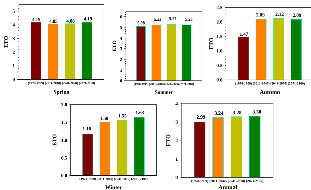
شکل (۵). میانگین سالانه و فصلی تبخیر و تعرق مرجع در دوره‌های مختلف تحت سناریوی RCP2.6 در ایستگاه سقز
