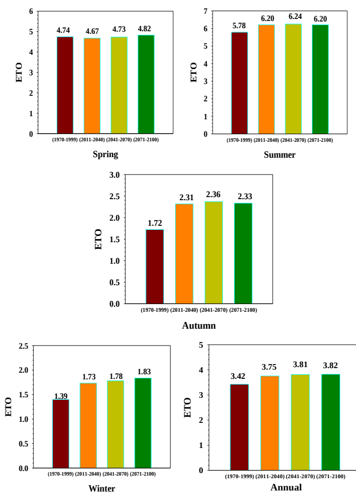
شکل (۳). میانگین سالانه و فصلی تبخیر و تعرق مرجع در دوره‌های مختلف تحت سناریوی RCP2.6 در ایستگاه سنندج
