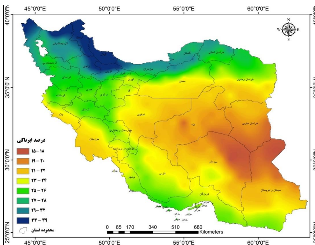
شکل (۳). میانگین درصد ابرناکی در پهنه ی ایران (۲۰۰۰-۲۰۱۰)
