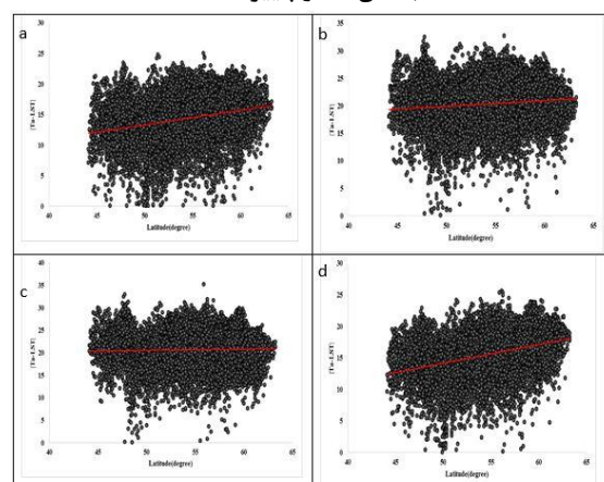
شکل (۷). نمودار پراکنش بین عرض جغرافیایی و قدر مطلق اختلافات دمای هوا و دمای سطح زمین در زمستان (a)، بهار (b)، تابستان (c) و پاییز (d).
