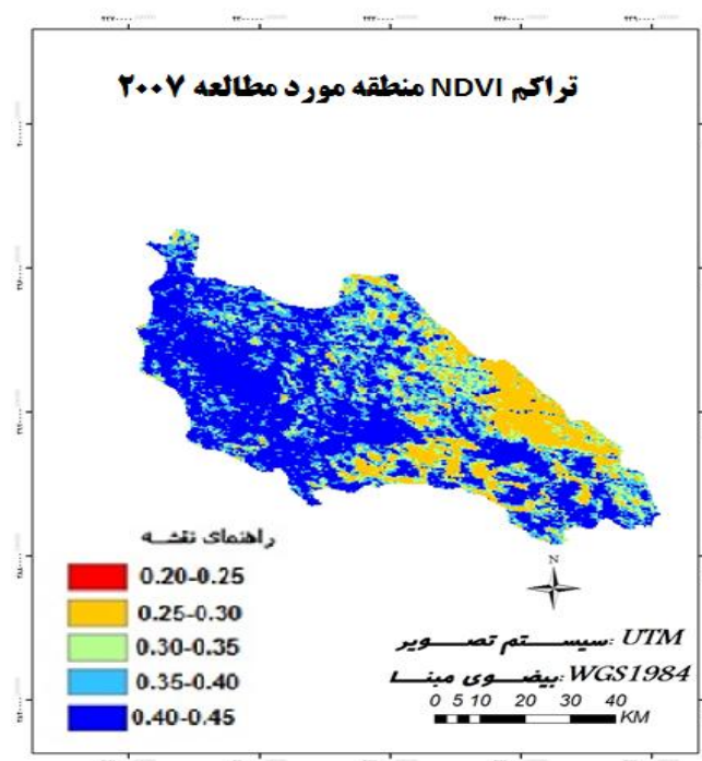
شکل (۷). میانگین NDVI ماه می منطقه مورد مطالعه سال ۲۰۰۷.
