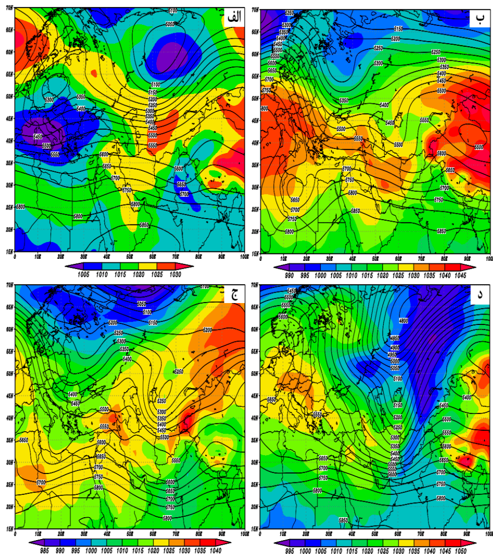
شکل (۳). نقشه ترکیبی فشار سطح دریا (نقشه رنگی) و آرایش توپوگرافی ارتفاع ژئوتانسیل تراز ۵۰۰ هکتوپاسکال (الف) روز ۱۲ دسامبر ۱۹۶۳ (طبقه امواج سرد ضعیف)، (ب) روز ۱۱ ژانویه ۱۹۸۳ (طبقه امواج سرد متوسط)، (ج) روز ۷ ژانویه ۱۹۸۹ (طبقه امواج سرد بسیار شدید)، (د) روز ۲۰ ژانویه ۱۹۶۴ (طبقه امواج سرد). ابر سرد).
