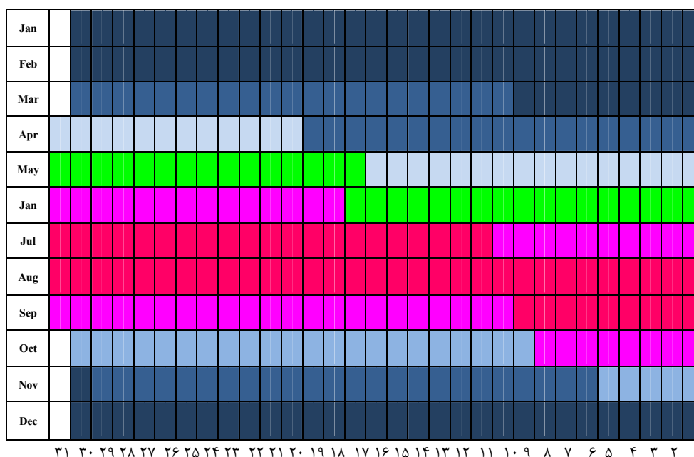
شکل (۳) طبقه بندی روزانه شاخص PMW بر حسب درجه تنش فیزیولوژیک در دریاچه گهر
