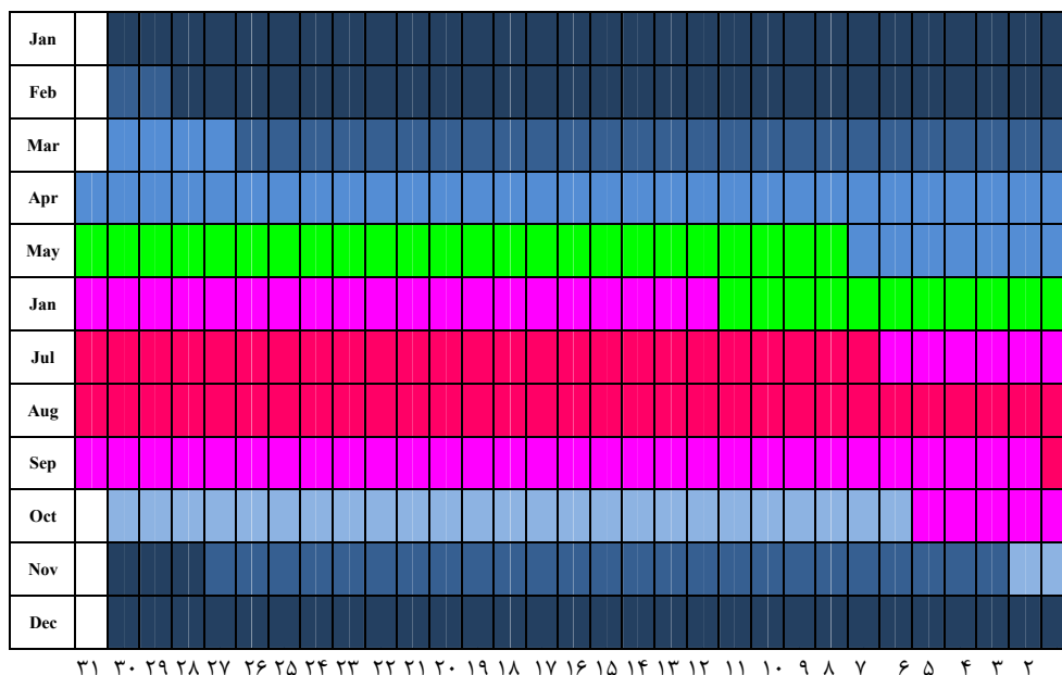
شکل (۲) طبقه بندی روزانه شاخص PET بر حسب درجه تنش فیزیولوژیک در دریاچه گهر (راهنمای شکل ۲ تا ۴)
