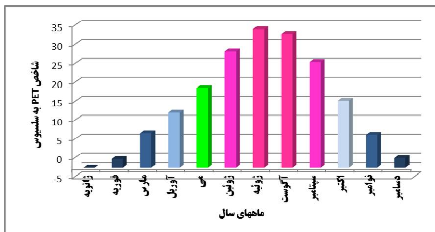
شکل (۵) طبقه بندی ماهانه شاخص های PET در دریاچه گهر
