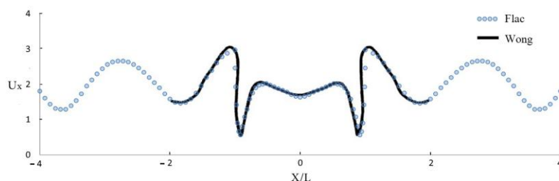
شکل ۱. صحت‌سنجی نتایج تحلیلی نرم‌افزار FLAC برای توپوگرافی دره ( R=25 , \lambda/R=2 ) موج قائم (SV)
