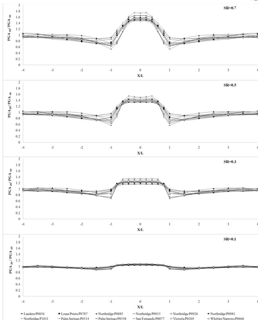
شکل ۹. نسبت نتایج بزرگ‌نمایی شتاب حاصل از تحلیل دوبعدی بر یک‌بعدی برای ۱۲ زلزله متفاوت با نسبت میرایی ۵٪ بر روی تپه‌ای با ضریب شکل‌های مختلف در فاصله‌های بی‌بعد شده از مرکز تپه
