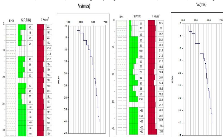
شکل ۵. پروفیل ژئوتکنیکی و ژئوفیزیکی گمانه ۴
