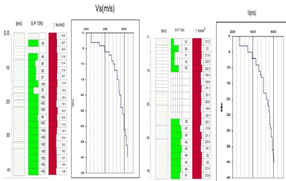
شکل ۳. پروفیل ژئوتکنیکی و ژئوفیزیکی گمانه ۲
