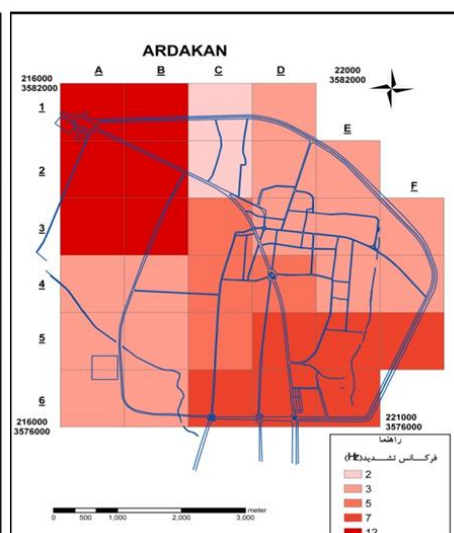
شکل ۱۲. نقشه توزیع فرکانس تشدید برای دوره بازگشت ۷۵ سال
