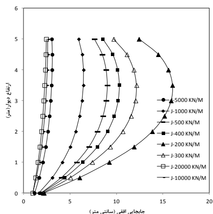
شکل ۱۲. نمودار جابه‌جایی افقی دیوار برای مقادیر مختلف سختی کششی مسلح‌کننده
