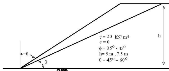
شکل ۵. شیب نمونه استفاده شده در تحلیل‌های لرزه‌ای
