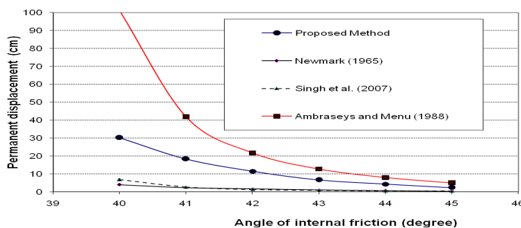
شکل ۱۲. مقایسه تغییر مکان ماندگار حاصل از روش‌های مختلف برای شیب مورد تحلیل
