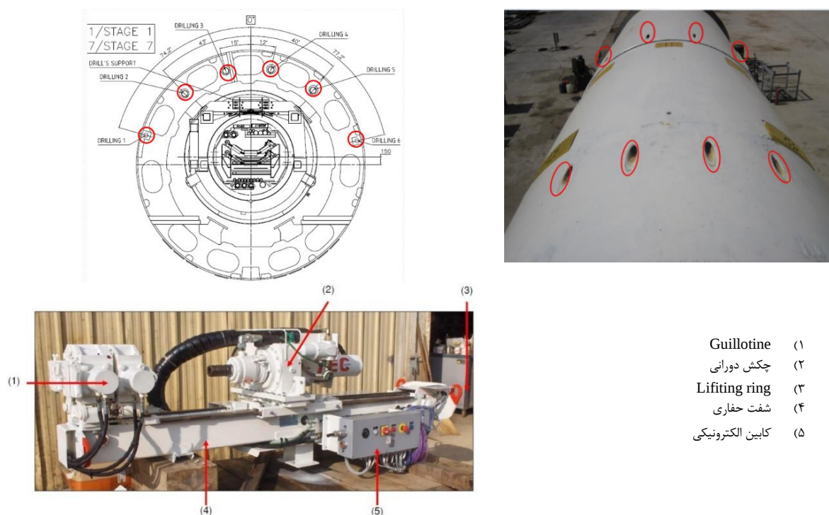
شکل ۹. مشخصه‌های سیستم حفاری پیشرو TBM
