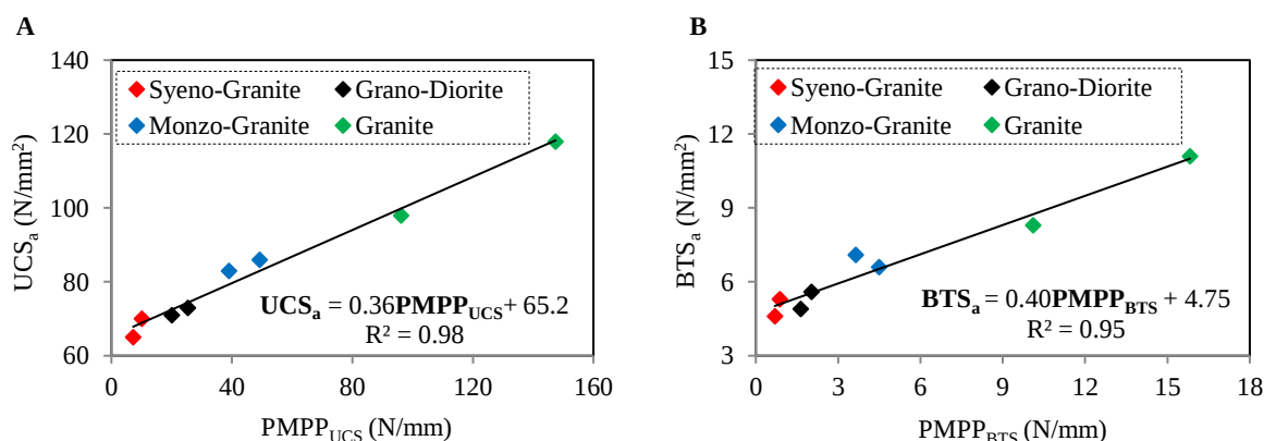
شکل ۱۴. رابطه دوام سنگ در برابر انجماد و آب شدن با پارامتر پترو-مکانیکی (A) مقاومت فشاری تک محوری (B) مقاومت کششی برزیلین نکته: دوام سنگ از طریق مقادیر مقاومت فشاری تک محوری ( UCS_a ) و مقاومت کششی برزیلین ( BTS_a ) بعد از فرایندهای انجماد و آب شدن ارزیابی شده است
