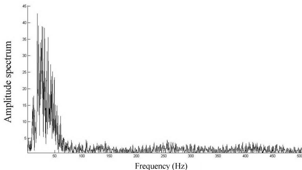
شکل ۹. طیف دامنه مربوط به رد لرزه‌ی سی‌ام شکل ۵ که از اعمال مرحله‌ی اول فیلتر میانی دو بعدی با طول پنجره‌ی ۹ نقطه به رکورد چشمه مشترک مصنوعی نوفه‌دار نشان داده شده در شکل ۳ به دست آمده و با استفاده از نرم‌افزار MATLAB ساخته شده است Fig. 9. The amplitude spectrum of thirtieth trace in Fig. 5 obtained from applying the first step of 2D median filter with 9 points window length on the indicated record in Fig. 3, and produced by MATLAB
