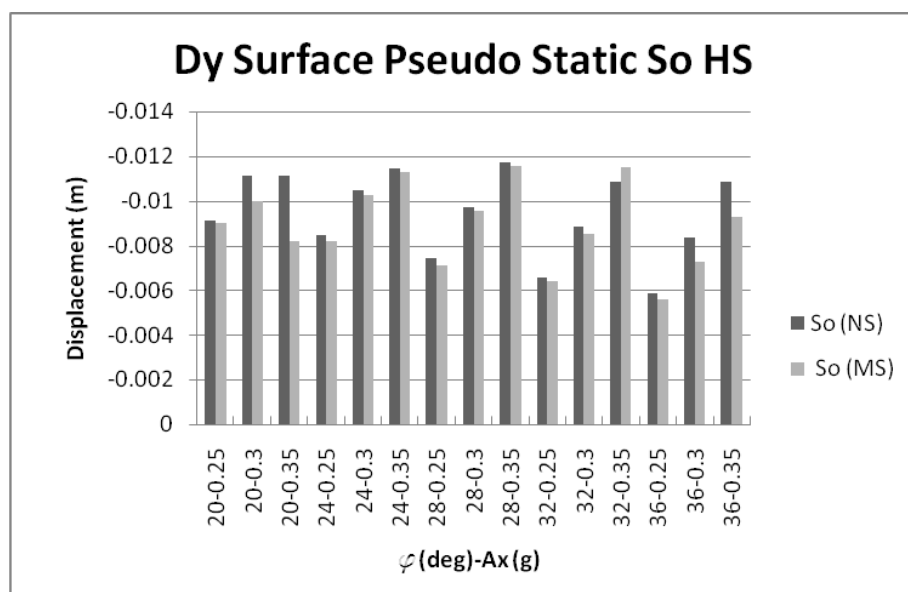
شکل ۵. تغییر مکان قائم سطح زمین در تحلیل‌های شبه استاتیکی با مدل رفتاری خاک سخت شونده برای خاک سست Fig. 5. Vertical displacement at the surface of the ground in pseudo static analyses with Hardening soil Model in soft soil
