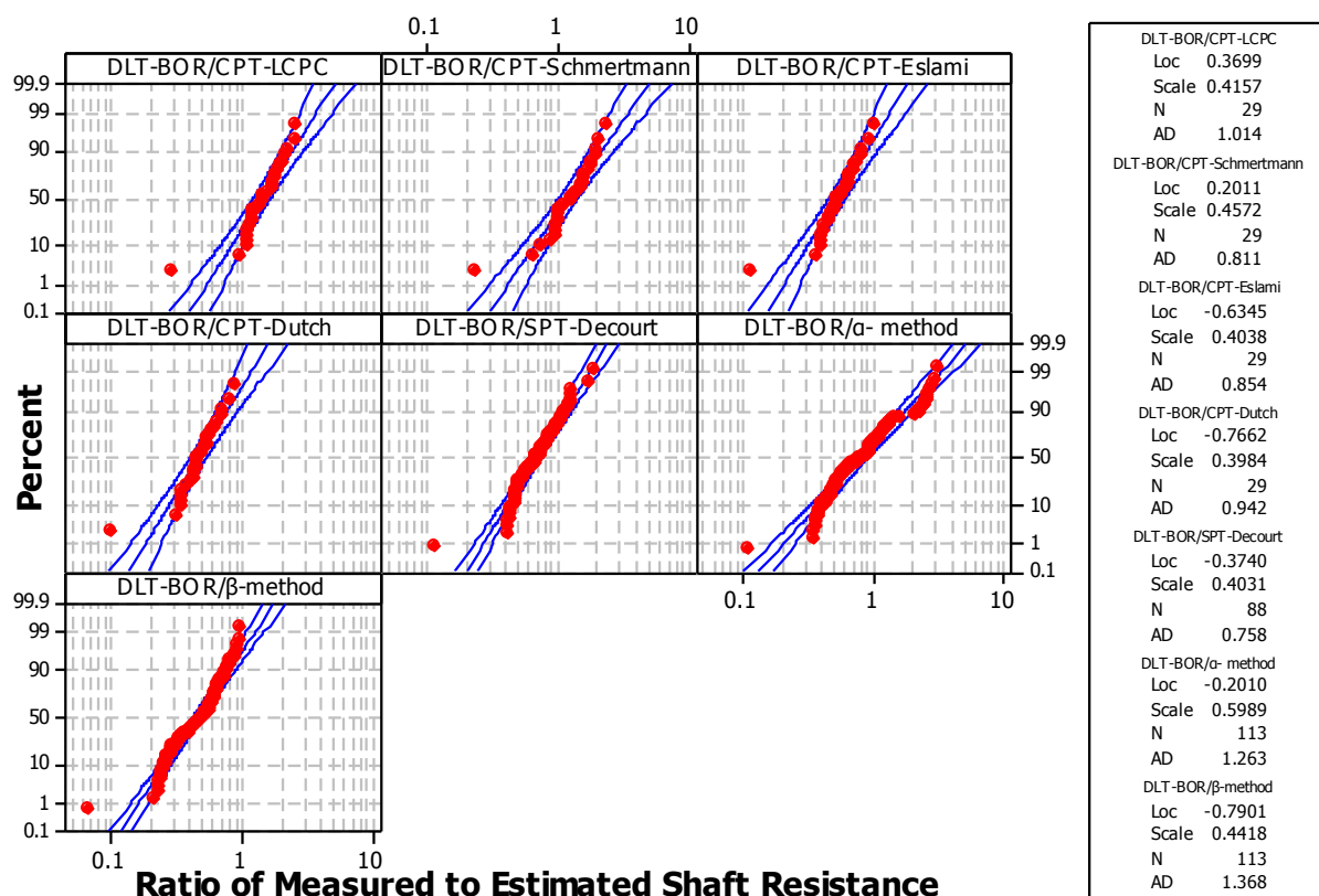
شکل ۳. نتایج آزمون AD برای ضرایب جهت گیری مقاومت جدار
