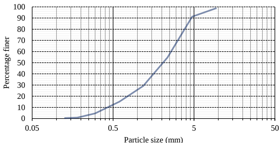
شکل ۱. منحنی دانه‌بندی سنگ‌دانه‌ها Fig. 1. Gradation curve of the aggregates
