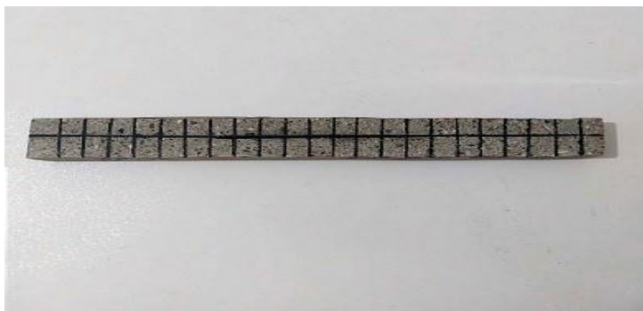
شکل ۵. شبکه‌بندی بر روی یک نمونه با سطح صیقلی
