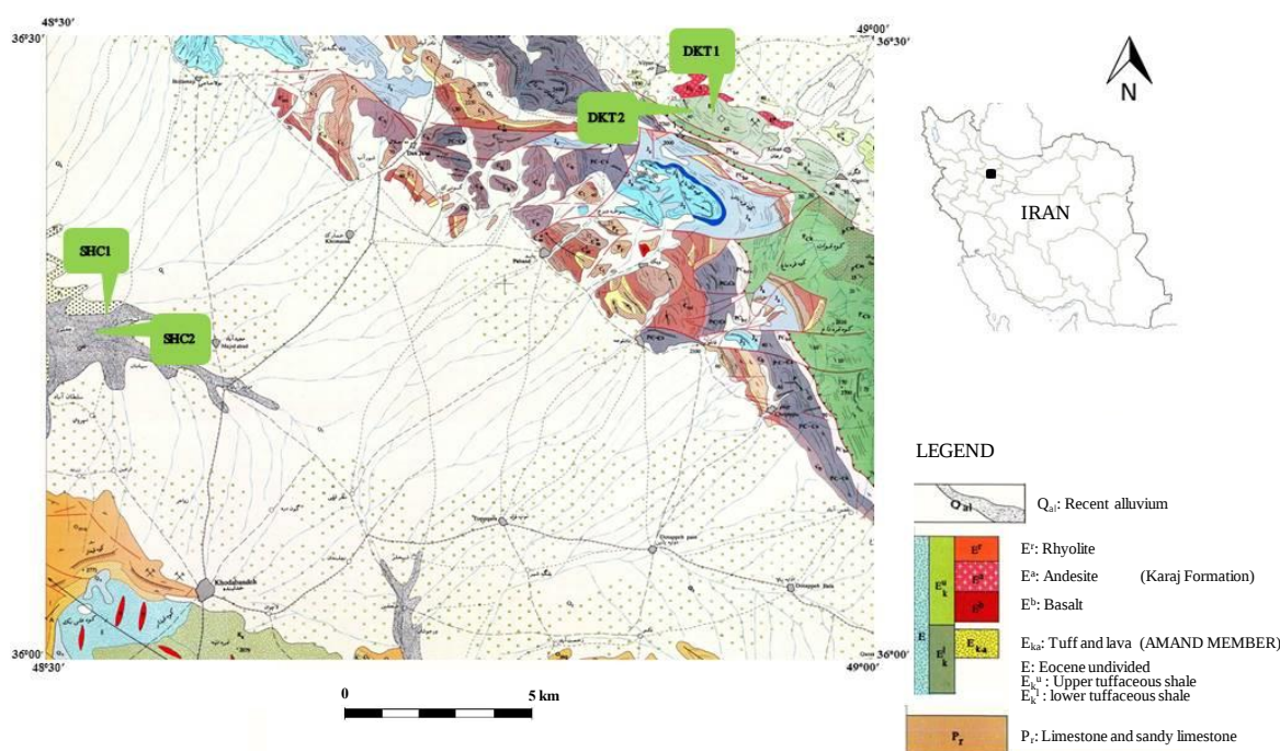
شکل ۲. موقعیت زمین‌شناسی منطقه و محل‌های نمونه برداری (هاشمی ۱۳۹۷) Fig. 2. Geological location of the region and sampling locations (Hashemi 1397)
