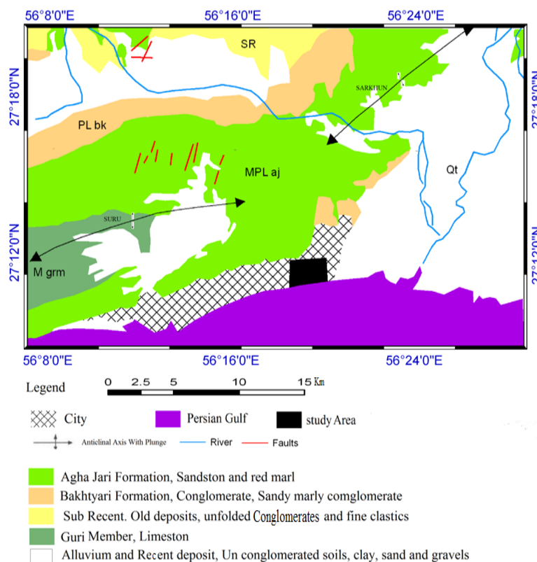
شکل ۲. نقشه زمین‌شناسی منطقه بستانو، برگرفته از نقشه ۱/۲۵۰۰۰ بندرعباس (فخاری، ۱۳۷۴)
