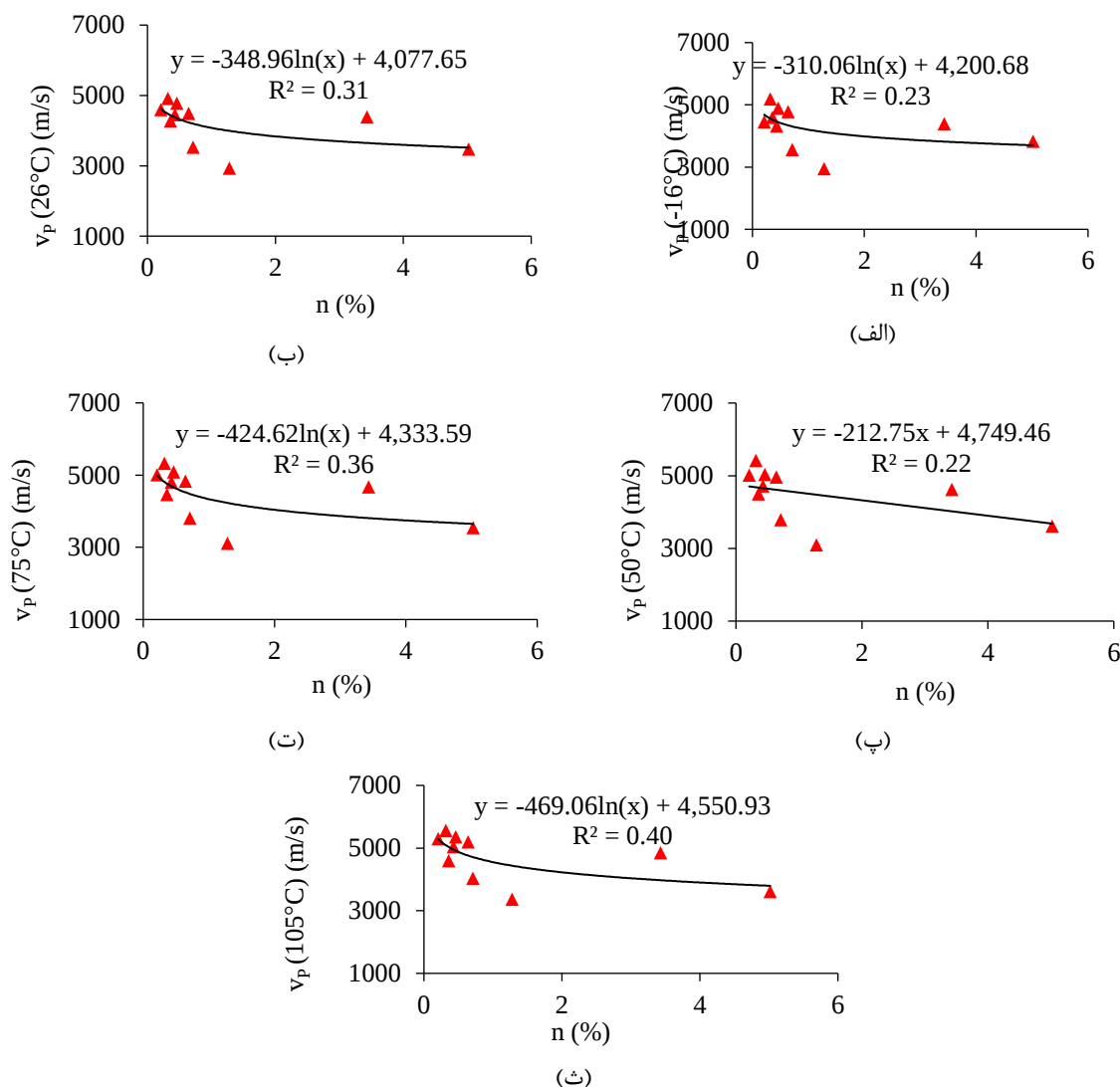
شکل ۴. ارتباط بین تخلخل و سرعت موج التراسونیک سنگ‌های مورد مطالعه در دماهای (الف) -16^{\circ}\text{C} ، (ب) 26^{\circ}\text{C} ، (پ) 50^{\circ}\text{C} ، (ت) 75^{\circ}\text{C} و (ث) 105^{\circ}\text{C} درجه سانتی‌گراد
