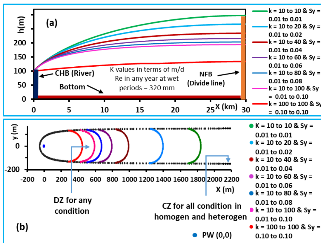
شکل ۹. اثر ناهمگنی: (a) سطح آب نرمال در پایان دوره‌ی تر. (b) حریم آبیگر و حریم تخلیه. خطوط زمان گذر یک ساله هستند. Fig. 9. The effect of heterogeneity: (a) Normal water level at the end of the wet period. (b) Capture Zone and Discharge Zone. Travel time lines are for 1 year.
