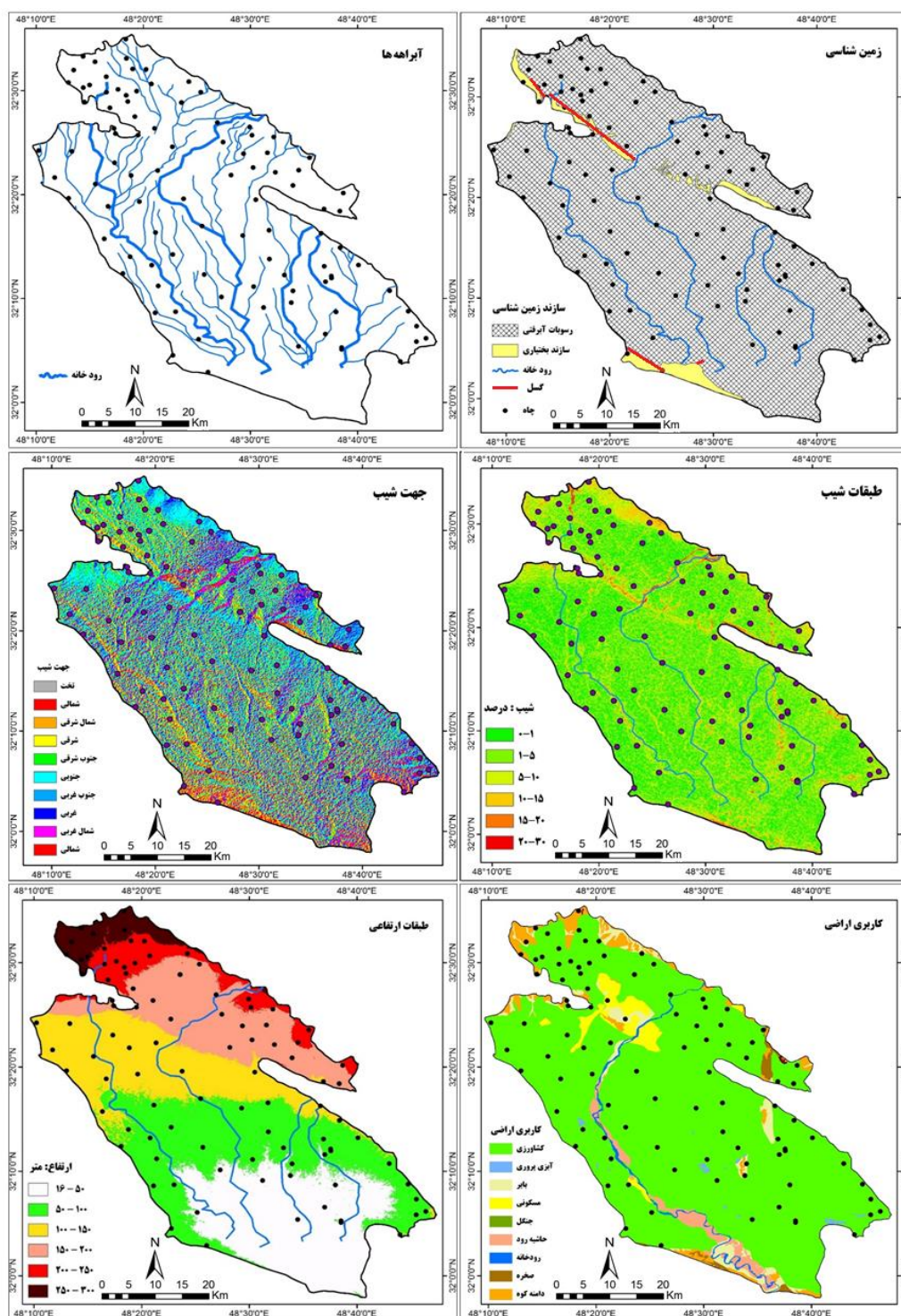
شکل ۲. نقشه‌های موضوعی دشت دزفول - اندیمشک
