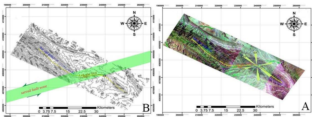
شکل ۵. A) نمودار امتداد سامانه‌های گسلی G1، G2 و G3 در بخش مرکزی منطقه مورد مطالعه (در پهنه گسل سررود در تاقدیس سررود)، B) محدوده پهنه گسلی سررود (محدوده سبز شده) و خمیدگی تاقدیس سررود در محل برخورد با ادامه جنوب غربی پهنه گسلی سررود (دید به سمت شمال غرب و تقریباً در راستای محور تاقدیس می‌باشد).
