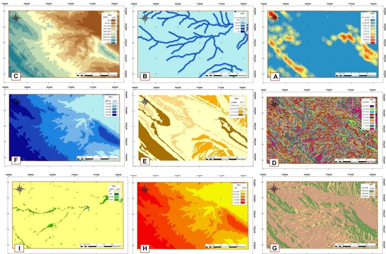
شکل ۱۰. نقشه‌های تهیه شده لایه‌های مؤثر در توسعه کارست در منطقه قره‌تیکان به روش سلسله مراتبی: A) درزه‌ها و شکستگی‌ها، B) فاصله از آبراهه‌ها، C) توپوگرافی (ارتفاعی)، D) شیب، E) لیتولوژی (سازندهای کربناته و غیرکربناته)، F) هم بارش، G) جهت شیب، H) هم دما، و I) کاربری اراضی (پوشش گیاهی).
