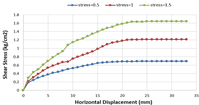
شکل ۲۵- نمودار جابجایی بر حسب تنش برشی نمونه شماره یک همراه با ۲۰٪ خرد بتن
