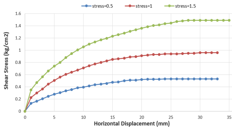
شکل ۲۷- نمودار جابجایی بر حسب تنش برشی نمونه شماره دو بدون وجود خرد بتن
