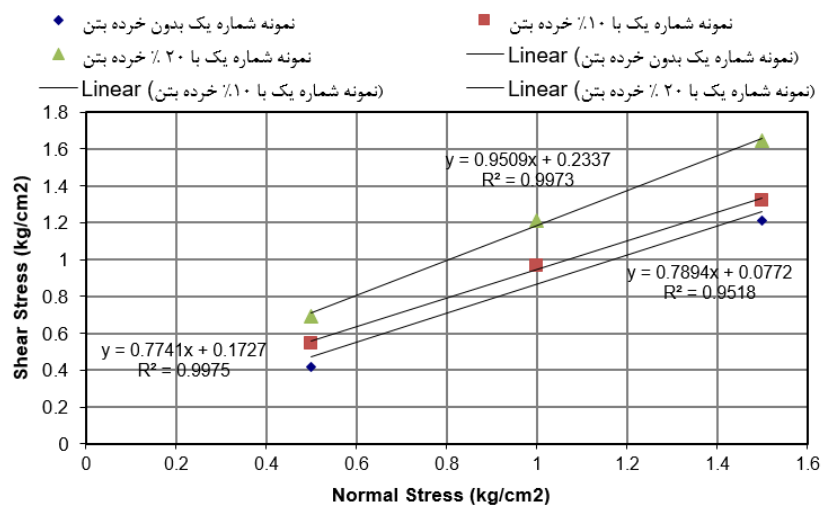
شکل ۲۶- پوش گسیختگی موهر کولمب نمونه شماره یک با و بدون حضور خرد بتن
