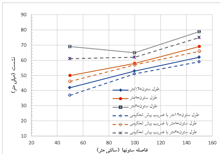
شکل ۱۵. مدل سازه خاکی با المان‌های تسلیح در سه حالت به طول‌های ۶، ۸ و ۱۲ متر
