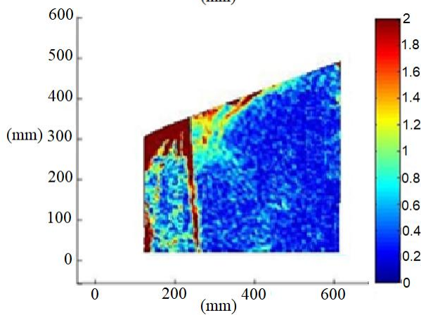
شکل ۹. کرنش برشی ایجاد شده در دیوار پایدارسازی شده با شیب پست ۲۰ درجه
