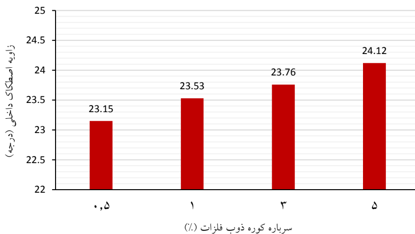
شکل ۱۵. تغییرات زاویه اصطکاک داخلی در مقابل مقدار سرباره کوره ذوب فلزات + ۲٪ آهک
