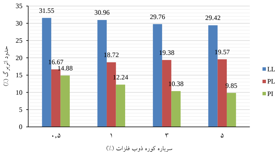
شکل ۲۴. مقایسه حدود اتربرگ و نشانه خمیری نمونه‌های با آهک ۱٪ و مقادیر مختلف سرباره
