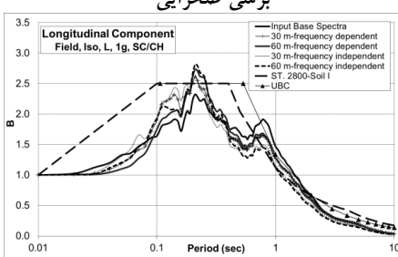
ه) PGA=1g خاک نوع I، مبنا سرعت موج برشی صحرایی
