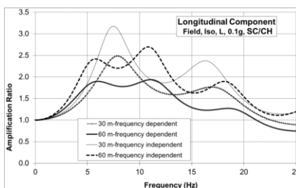
الف) PGA=0.1g خاک نوع I، مبنا سرعت موج برشی صحرایی
