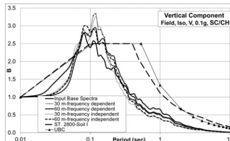
الف) PGA=0.1g ، خاک نوع I، مبنا سرعت موج برشی صحرایی
