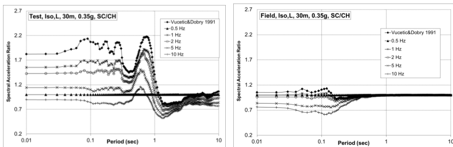
الف) ستون ۳۰ متری خاک نوع I، مینا سرعت موج برشی صحرایی ب) ستون ۳۰ متری خاک نوع IV، مینا سرعت موج برشی آزمایشگاهی شکل ۹. متوسط تغییرات نسبت شتاب طیفی مؤلفه L زلزله‌های میدان نزدیک ( PGA=0.35g ) به شتاب طیفی مصالح با فرکانس بارگذاری ۰/۵
