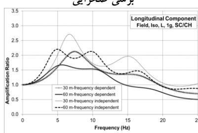
ه) PGA=1g خاک نوع I، مبنا سرعت موج برشی صحرایی
