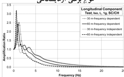
ی) PGA=1g خاک نوع IV، مبنا سرعت موج برشی آزمایشگاهی
