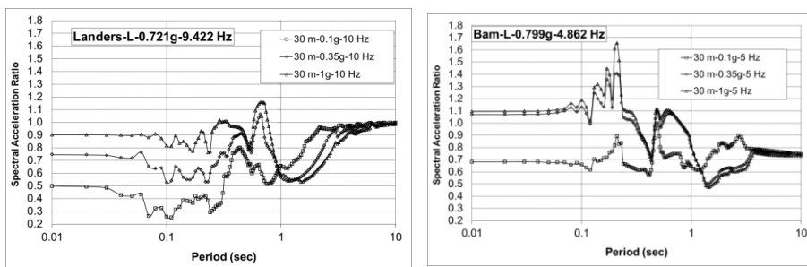
الف) زلزله بم با فرکانس غالب ۴/۹ Hz ب) زلزله لندرز (رکورد LCN) با فرکانس غالب ۹/۴ Hz
