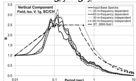
ه) PGA=1g ، خاک نوع I، مبنا سرعت موج برشی صحرایی
