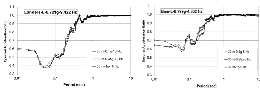
الف) زلزله بم با فرکانس غالب 4/9 Hz ب) زلزله لندرز (رکورد LCN) با فرکانس غالب 9/4 Hz
