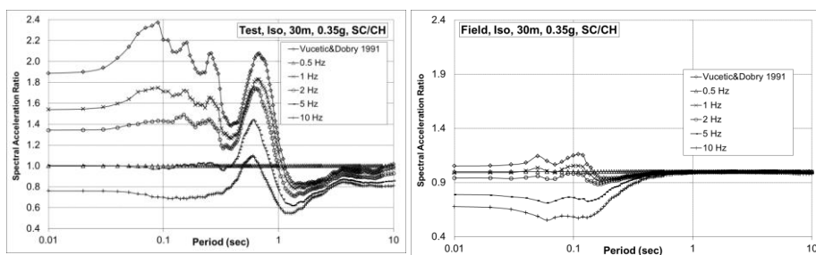
الف) ستون ۳۰ متری خاک نوع I، مینا سرعت موج برشی صحرایی ب) ستون ۳۰ متری خاک نوع IV، مینا سرعت موج برشی آزمایشگاهی شکل ۱۰. متوسط تغییرات نسبت شتاب طیفی هر سه مؤلفه زلزله‌های میدان نزدیک ( PGA=0.35g ) به شتاب طیفی مصالح با فرکانس بارگذاری ۰/۵ Hz
