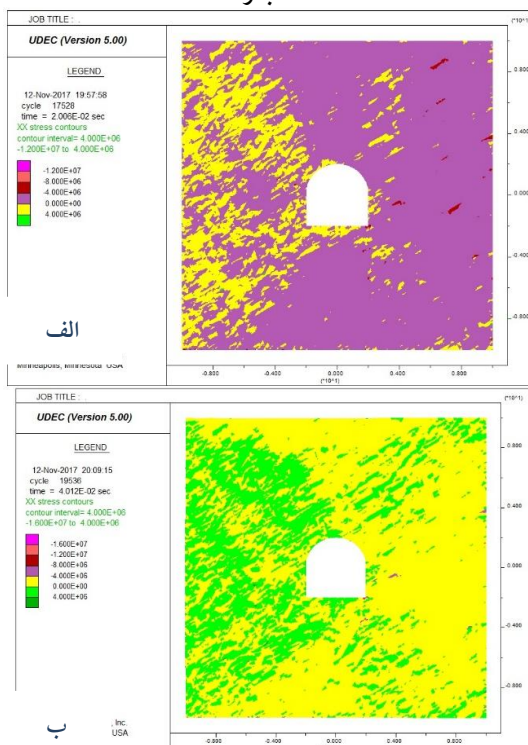
شکل ۱۳. کنتور تنش در راستای x ( S_{xx} ) در اطراف رمپ در مدت زمان الف) ۲۰ میلی ثانیه، ب) ۴۰ میلی ثانیه از اعمال بار دینامیکی انفجار
