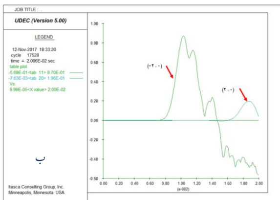
شکل ۱۲. تاریخچه زمانی سرعت‌های افقی در نقاط شاهد (-2, 0) و (2, 0) روی دیواره سمت چپ و راست رمپ در مدت زمان الف) ۲۰ میلی ثانیه، ب) ۴۰ میلی ثانیه از اعمال بار دینامیکی انفجار
