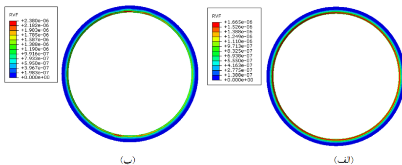
شکل ۶. مقایسه دبی نشست آب از تونل در دو توزیع میلگرد؛ الف) ۲۰ cm @ \Phi 16 \text{ mm} و ب) ۳۰ cm @ \Phi 20 \text{ mm}
