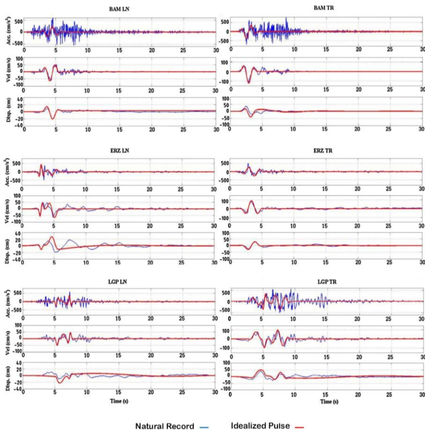
شکل ۱۳. تاریخچه زمانی شتاب، سرعت و جابه‌جایی متناظر با رکوردهای BAM، ERZ و LGP (جدول ۱) و ساختار ریاضی مدل فرم بسته معادل
