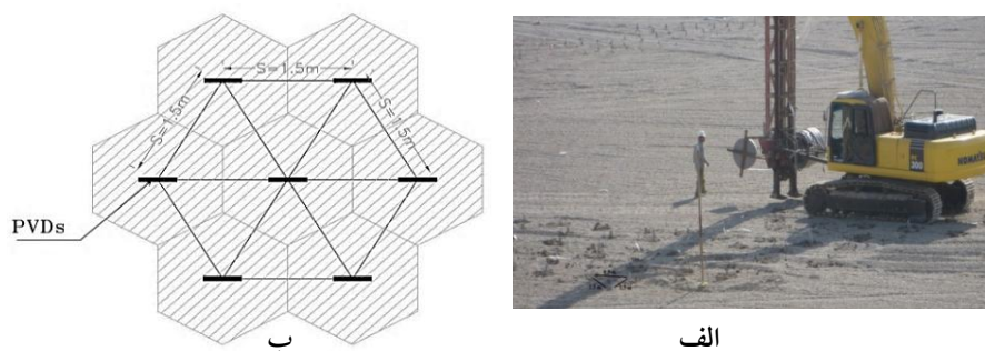
شکل ۶. الف) نمای از اجرای زهکش‌های نواری در زیر خاکریزها، ب) آرایش زهکش‌ها در پلان
