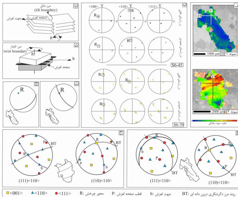
شکل ۵. مراحل شناسایی سیستم‌های لغزشی فعال در بلورهای نمک به روش تحلیل دگرشکلی پدیدار شده در دانه‌ها. توضیح قسمت‌های الف تا ج در متن ارائه شده است. در قسمت‌های ج و چ، دایره عظیمه خط چین معرف مرز دگرشکلی درون دانه، دایره عظیمه توپر معرف سطح لغزش، نماد ( ) معرف صفحه و نماد < > معرف محور بلورشناسی است.
