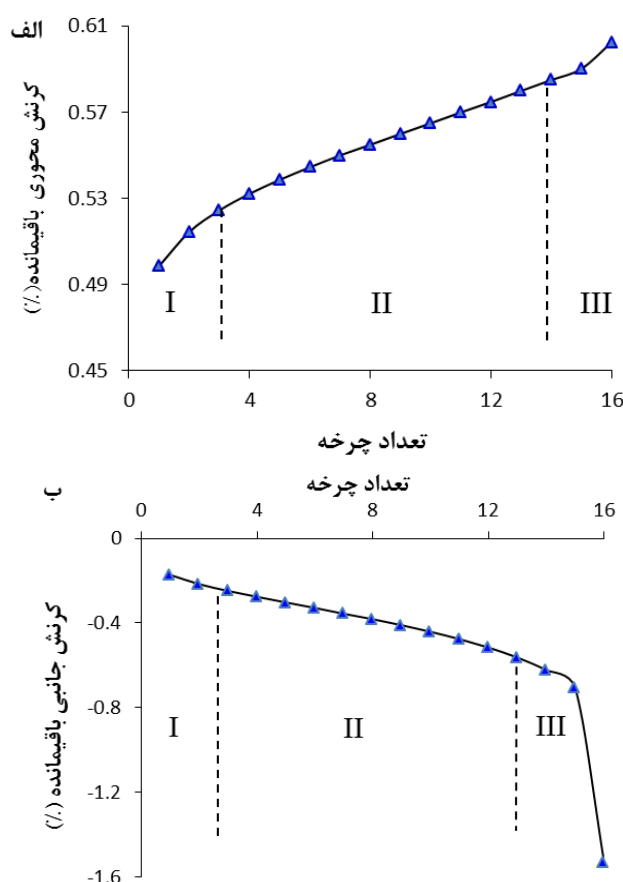
شکل ۵. روند تغییرات سه مرحله‌ای کرنش‌های باقی‌مانده (الف) محوری و (ب) جانبی (نمونه T05) نکته قابل توجه در روند تغییرات کرنش محوری افزایش شدید این پارامتر در چرخه اول نسبت به سایر چرخه‌ها است. این مطلب می‌تواند ناشی از بسته شدن ناپیوستگی‌های موجود در نمونه و همچنین به دلیل بارگذاری آرام تا تراز تنش متوسط باشد. برخلاف روند تغییرات کرنش محوری، تشخیص فاز توسعه شتاب‌دار ترک در روند تغییرات کرنش جانبی، امکان‌پذیر است. این امر ناشی از این حقیقت است که ترک‌ها عمدتاً در راستای بارگذاری ایجاد شده و باعث شده‌اند که این پارامتر به بارگذاری چرخه‌ای حساس‌تر باشد. چنان‌که در شکل‌های ۶ و ۷ دیده می‌شوند، ضعیف‌شوندگی پیش‌رونده باعث شده تا با افزایش تعداد چرخه‌ها، اختلاف بین کرنش‌های حداکثر و باقی‌مانده افزایش یابد.
