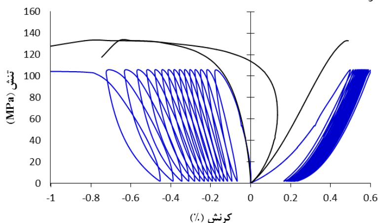
شکل ۴. منحنی تنش کرنش استاتیکی و دینامیکی برای توانالیت الوند (نمونه T05)
