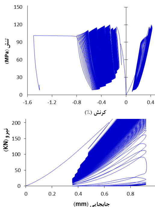
شکل ۱۳. روند تغییرات نیرو-جابجایی دستگاه اینسترون و تغییرات تنش-کرنش طی آزمایش خستگی جابه‌جایی کنترل (نمونه T03)
