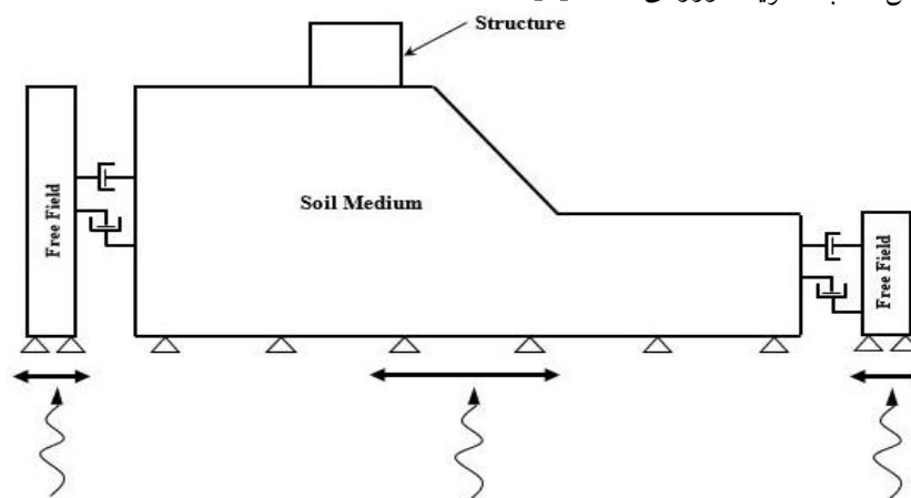
شکل ۵. مدل المان محدود سیستم خاک-سازه و شبیه‌سازی مرزهای جانبی به‌کار رفته در آنالیزها ۲. مدل‌سازی عددی
