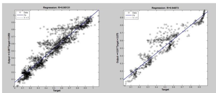
شکل ۱۱. نمودار ضریب هم‌بستگی در مرحله آزمون در روش RBF
