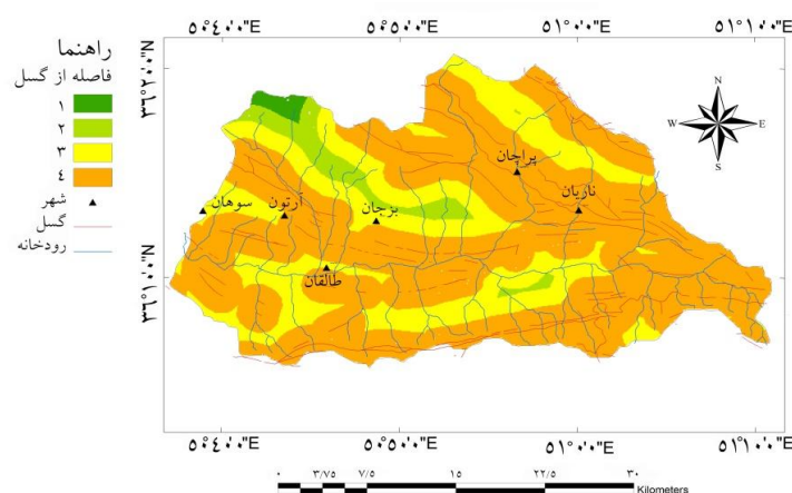
شکل ۷. نقشه فاصله از گسل رتبه داده شده منطقه طالقان
