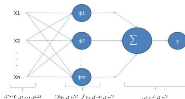
شکل ۳. ساختار کلی از شبکه‌های عصبی مبتنی بر توابع پایه‌ای گوسی
