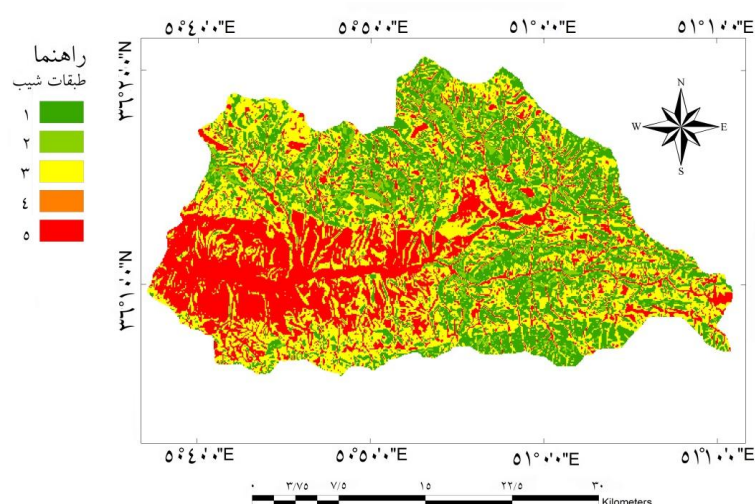
شکل ۶. نقشه شیب رتبه داده شده منطقه طالقان
