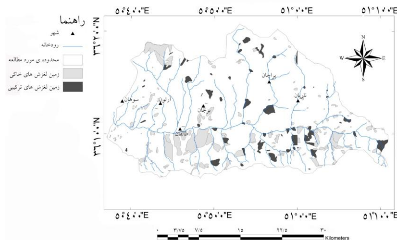
شکل ۵. نقشه پراکندگی محدوده کل لغزش‌های خاکی و ترکیبی (خاکی و سنگی) موجود در محدوده بررسی شده (بانک اطلاعاتی زمین‌لغزش‌های کشور، سازمان جنگل‌ها، مراتع و آبخیزداری کل کشور)
