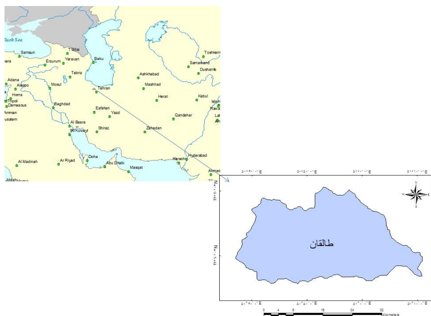
شکل ۱. موقعیت منطقه بررسی شده
