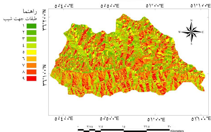
شکل ۷. نقشه جهت شیب رتبه داده شده منطقه طالقان
