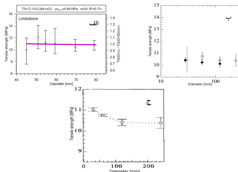
شکل ۱. پژوهش‌های انجام شده در زمینه تأثیر قطر نمونه بر مقاومت کششی برزیلی؛ الف) پژوهش‌های گوبینی و همکاران [۳۹] روی نمونه‌های گرانیتی، ب) پژوهش‌های روکو و همکاران [۱۴] روی نمونه‌های گرانیتی، ج) پژوهش‌های تورو و همکاران [۴۲] روی نمونه‌های سنگ آهک
