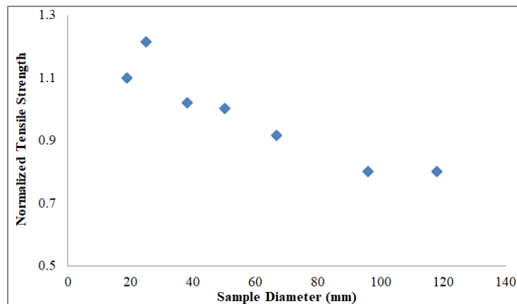
شکل ۹. تأثیر قطر نمونه بر مقاومت کششی نرمالیزه شده نسبت به قطر ۵۰ میلی‌متر
