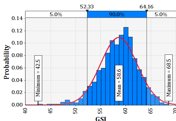
شکل ۹. تابع توزیع GSI حاصل از فرمول کای و کایزر و شبیه‌سازی مونت کارلو (درزه‌های منظم و غیرمداوم)
