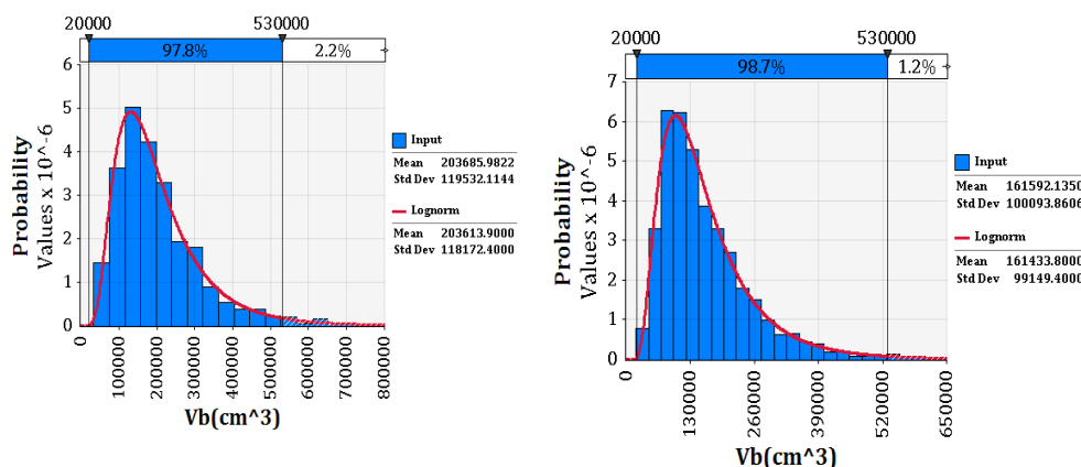
شکل ۴. توزیع حجم بلوک‌ها با فرض سه دسته درزه مداوم شکل ۵. توزیع حجم بلوک‌ها با فرض وجود درزه‌های غیرمداوم
