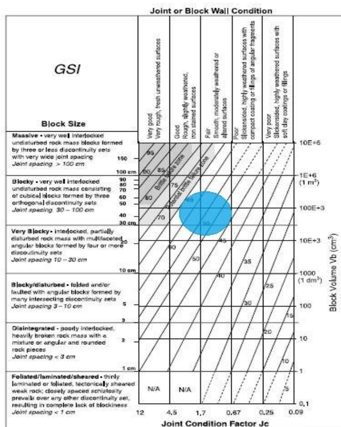
شکل ۲. نمودار کمی GSI ارائه شده به وسیله کای و همکاران (۲۰۰۴) [۹] جدول ۱. جهت‌داری ناپیوستگی‌های موجود در تکیه‌گاه چپ سد بختیاری [۱۲]
