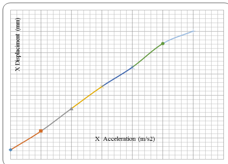
شکل ۱۶. نمودار اثر شتاب ثقل افقی زمین بر جابه‌جایی افقی زمین در شيروانی کمروء.
