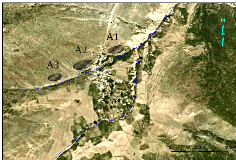
شکل ۴. عکس ماهواره ای از منطقه که در آن سه رخنمون سنگی برداشت شده مشخص شده است
