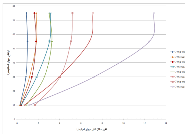
شکل ۸. تأثیر نحوه اجرای تسمه‌های پلیمری بر تغییر مکان دیوار
