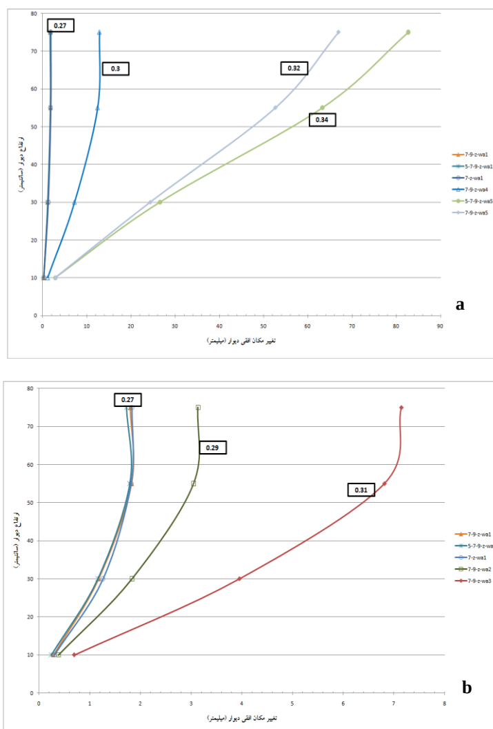
شکل ۱۵. محدوده تغییرات ضرایب شتاب افقی معادل زلزله برای مدل (k'_h) در دیوارهای خاک مسلح شده با اجرای زیگزاکی تسمه‌های پلیمری، (a) اثر تغییر بیشینه شتاب موج ورودی، (b) اثر تغییر فرکانس
