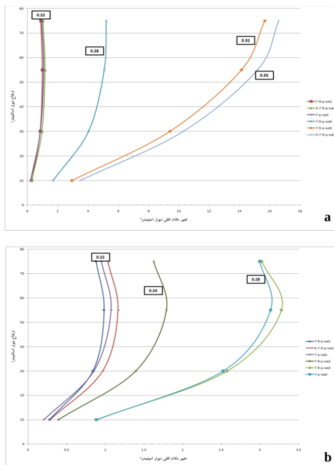
شکل ۱۴. محدوده تغییرات ضرایب شتاب افقی معادل زلزله برای مدل ( k'_h ) در دیوارهای خاک مسلح شده با اجرای موازی تسمه‌های پلیمری، (a) اثر تغییر بیشینه شتاب موج ورودی، (b) اثر تغییر فرکانس
